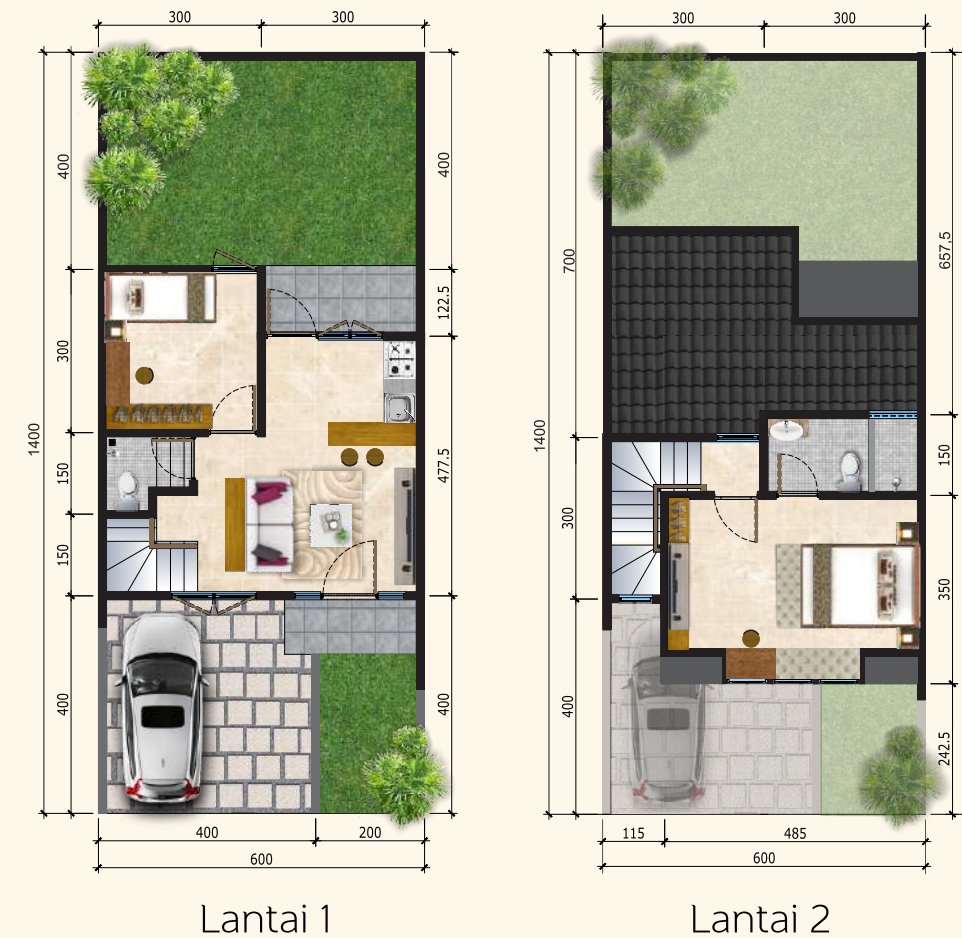
MONTERREY 2B (Kavling 6x14m | LB.61/LT.84)
